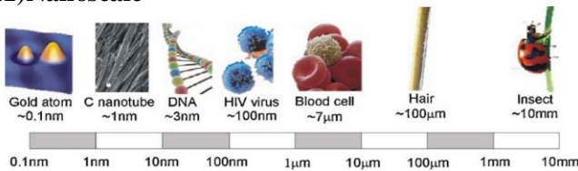
Figure 1.1. Nanoscale
